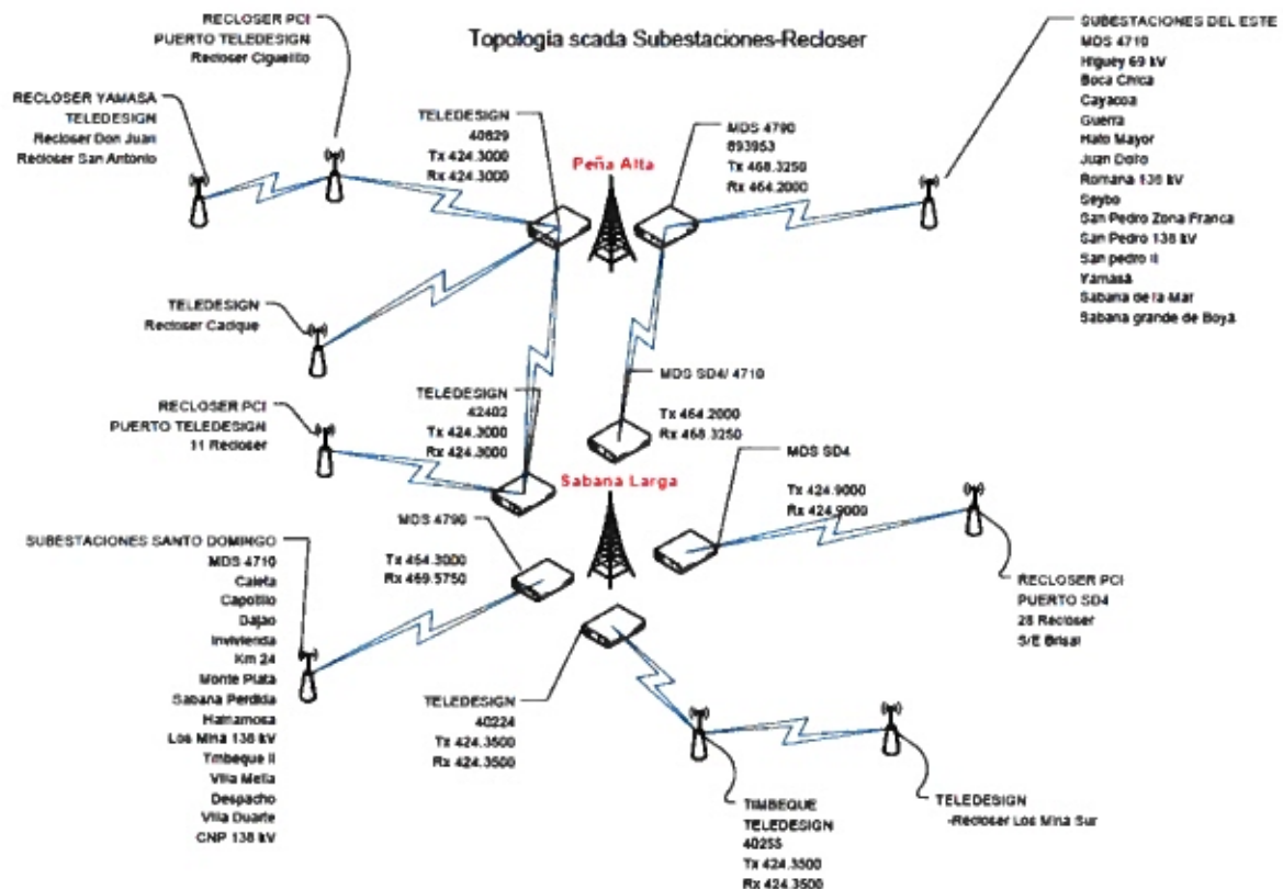
Diagrama general de la red de Scada conexión subestaciones-Recloser EDE Este
